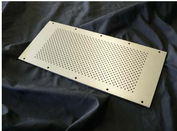
Laserzuschnitt, t=5mm inkl. 130 Rundlöcher \varnothing=3\text{mm}
